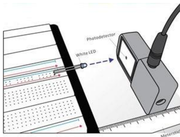
Skúmanie osvetlenia v závislosti od vzdialenosti od zdroja svetla
