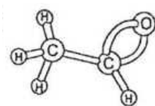
Acetaldehyd
