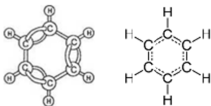
Benzén
