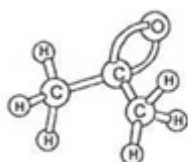
Dimetylketón (acetón)
