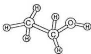
Etanol
