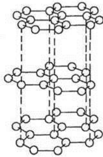
Grafit
