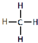
CH 4
