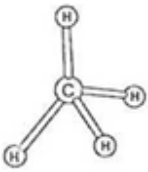
Metán
