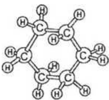
Cyklohexán
