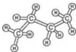
Bután
