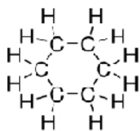
C 6 H 12
